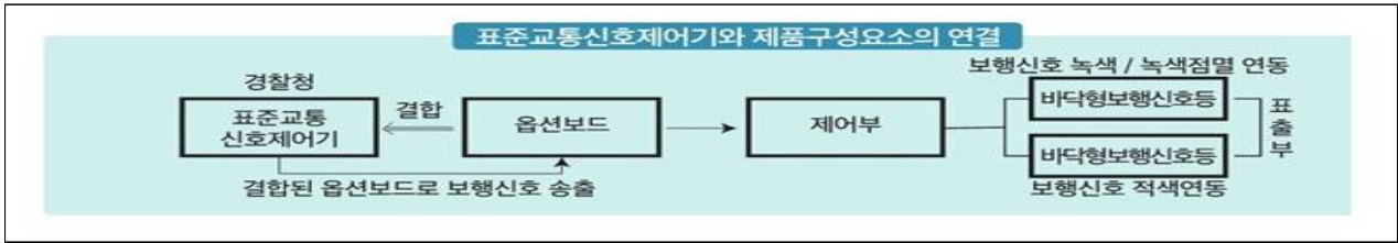
[그림 2] 표준교통신호제어기와 바닥형 보행신호등 구성도
